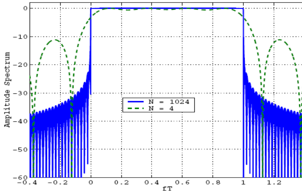
Φάσματα OFDM σημάτων, με 4 και με 1024 υποφέροντα.
