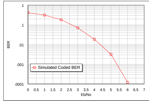
BPSK
