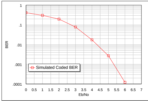
QPSK
