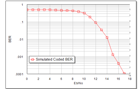
256QAM
