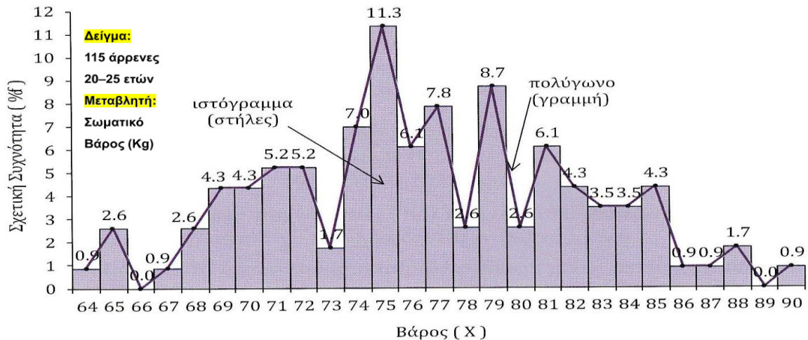
Σχήμα 3.2 - Ιστογράμμα και πολύγωνο σχετικής συχνότητας (%f) της απλής κατανομής του Βάρους (N = 115)
