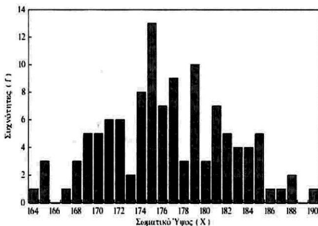
Εικ. 3.1 - Ιστογράμμα συχνοτήτων κατανομής (N=115)
