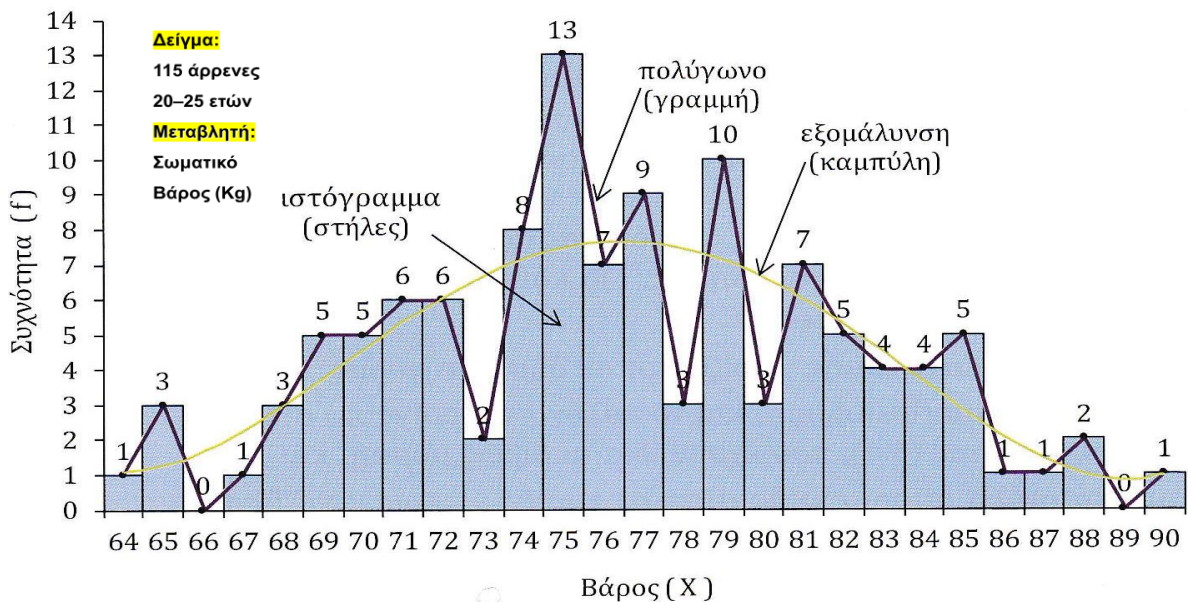
Σχήμα 3.1 - Ιστόγραμμα και πολύγωνο συχνότητας ( f ) της απλής κατανομής του Βάρους ( N = 115 )
