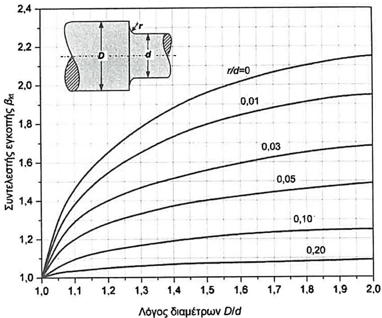
ΔΙΑΓΡΑΜΜΑ 4: Συντελεστής εγκοπής \beta_{Kt} για άτρακτο με διαβάθμιση και καταπόνηση σε στρέψη (αντοχή χάλυβα \sigma_B = 700 \text{ N/mm}^2 )
