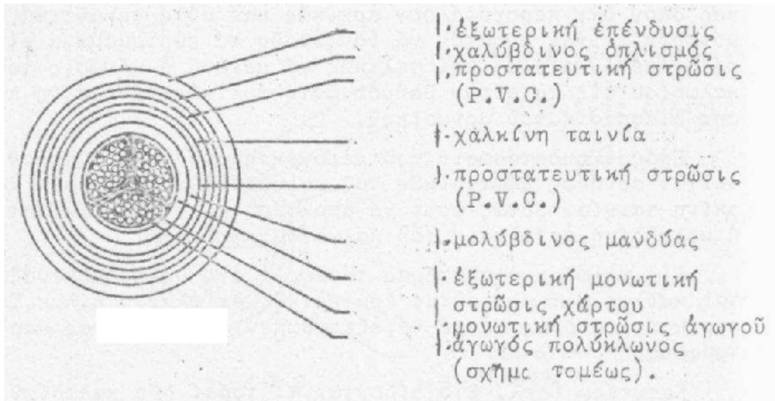
ΜΟΝΟΠΟΛΙΚΑ ΚΑΛΩΔΙΑ ΜΤ ΜΕ ΜΟΝΩΣΗ ΧΑΡΤΙ
