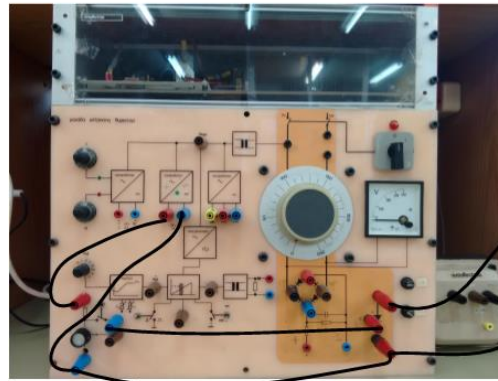
Κύκλωμα Μέτρησης Ρεύματος Συγκράτησης-Διατήρησης
