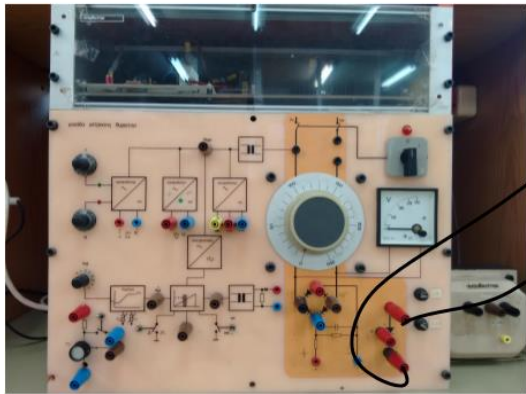
Κύκλωμα Αρνητικής Αποκοπής
