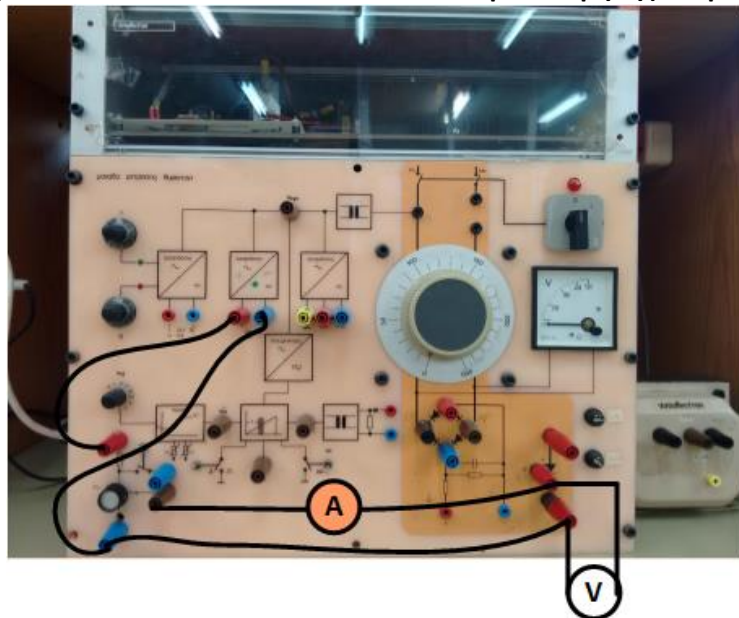
Κύκλωμα Χαρακτηριστικής Πύλης - Καθόδου
