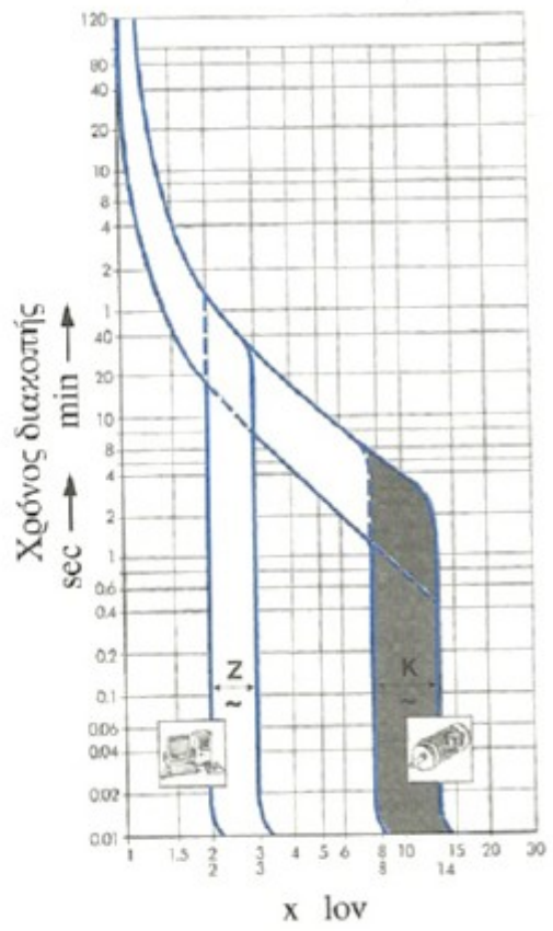
Χαρακτηριστικές καμπύλες Z, K EN 60947-2, IEC 947-2
