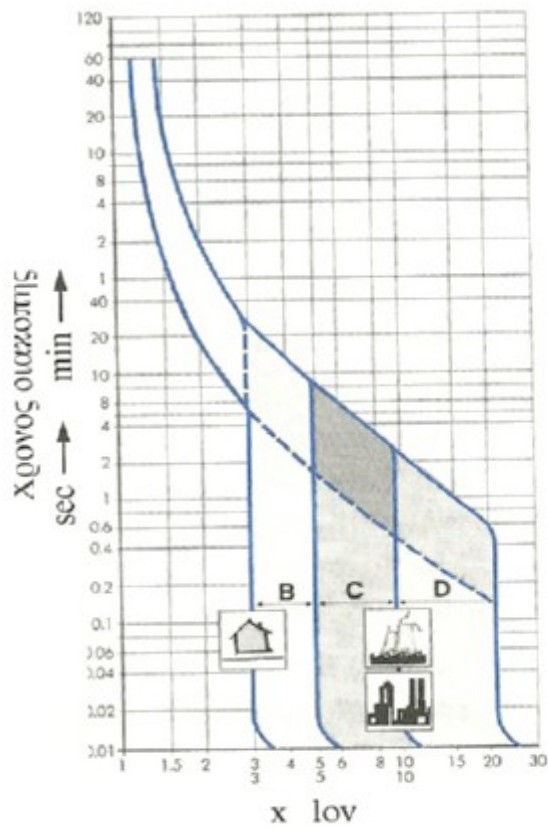
Χαρακτηριστικές καμπύλες B, C, D EN 60898, IEC 896
