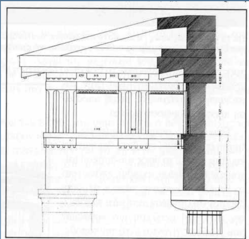
Εικ.15 Μερική αναπαράσταση της όψεως του "κτηρίου Η" (Wiegand)
