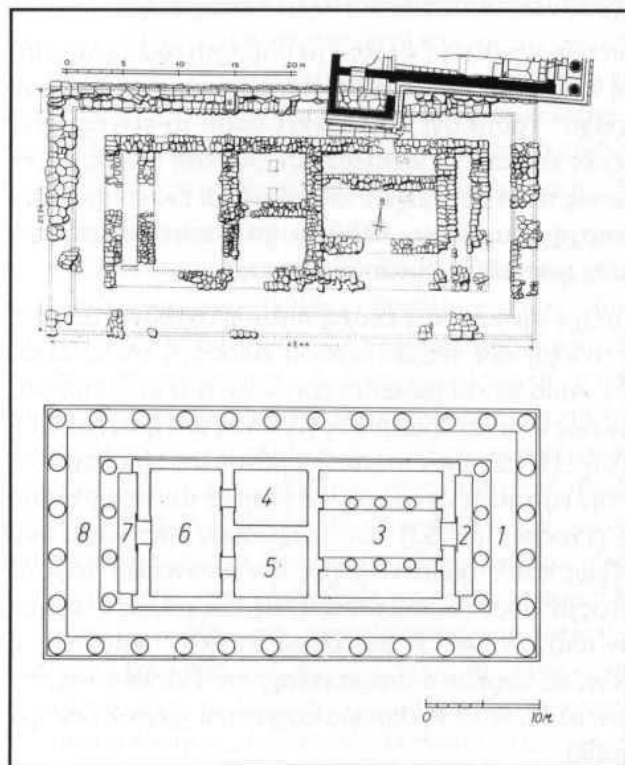
Εικ.10 Άνω. Τα θεμέλια του αρχαίου νεώ (Dörpfeld). Κάτω. Αναπαράσταση της κατόψεως του 'αρχαίου νεώ: 1. ανατολικό πτερόν, 2. ανατολική πρόστασις, 3. ανατολικό διαμέρισμα (ιερόν της Αθηνάς), 4-5-6. δυτικό διαμέρισμα (οπισθοδόμος), 4. αριστερό δωμάτιο οπισθοδόμου, 5. δεξιό δωμάτιο οπισθοδόμου, 6. προθάλαμος οπισθοδόμου, 7. δυτική πρόστασις, 8. δυτικό πτερόν
