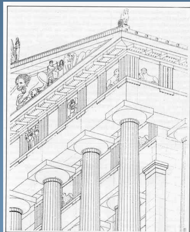
Εικ. 19 Αναπαράσταση της ΒΑ γωνίας του 'κτηρίου Η' (πρωταρχικός Παρθενών) Ο σκόκος παρίσταται ως δίστυλος εν παραστάσει, είναι, όμως, εξ ίσου πιθανόν ότι ήταν τετράστυλος πρόστυλος. Το γωνιαίο ακρωτήριο παρίσταται στην πρώτη, μετά την ανανέωση του βάθρου, μορφή. Το πρωταρχικό ακρωτήριο (ή έλιξ) συνυπάρχει με το νέο. Το κορυφαίο ακρωτήριο παρίσταται ανανεωμένο για δεύτερη φορά (αλλαγή προγενεστέρου ανθεμίου ή γλυπτού και προσθήκη κορών εκατέρωθεν). Από την πρώτη ανανέωση παραμένει μόνον ο κεντρικός λίθος του βάθρου. Από το πρωταρχικό ακρωτήριο (Γοργώ) παραμένουν μόνον κατάλοιπα του μικρού υποβάθρου του κάτω από το πολύ μεγαλύτερο νέο βάθρον.
