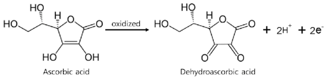
Εικόνα 1. Οξειδωτικές καταστάσεις ασκορβικού οξέος
