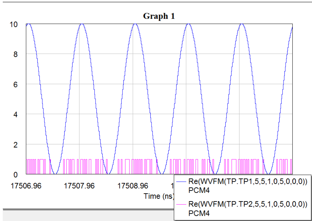
Εικόνα 11 – Κωδικοποίηση σήματος
