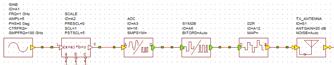
Εικόνα 10: PCM εκπομπός
