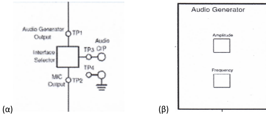
Εικόνα 4 – (α) Μονάδα επιλογής σήματος εισόδου, (β) Κομβία καθορισμού συχνότητας και πλάτους στη γεννήτρια ακουστικού σήματος
