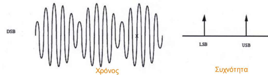
Εικόνα 6 – AM διαμόρφωση (πεδίο χρόνου και πεδίο συχνότητας)
