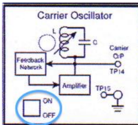
Εικόνα 7 – Βαθμίδα Carrier Oscillator στο IT-4101 board
