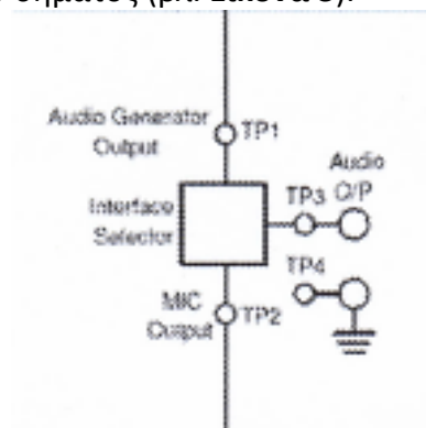
Εικόνα 3 – Μονάδα επιλογής σήματος εισόδου στο IT-4101 board
