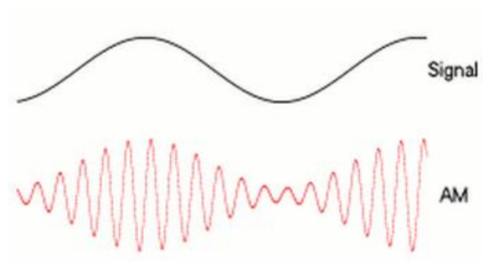
Εικόνα 1 – Η AM διαμόρφωση
