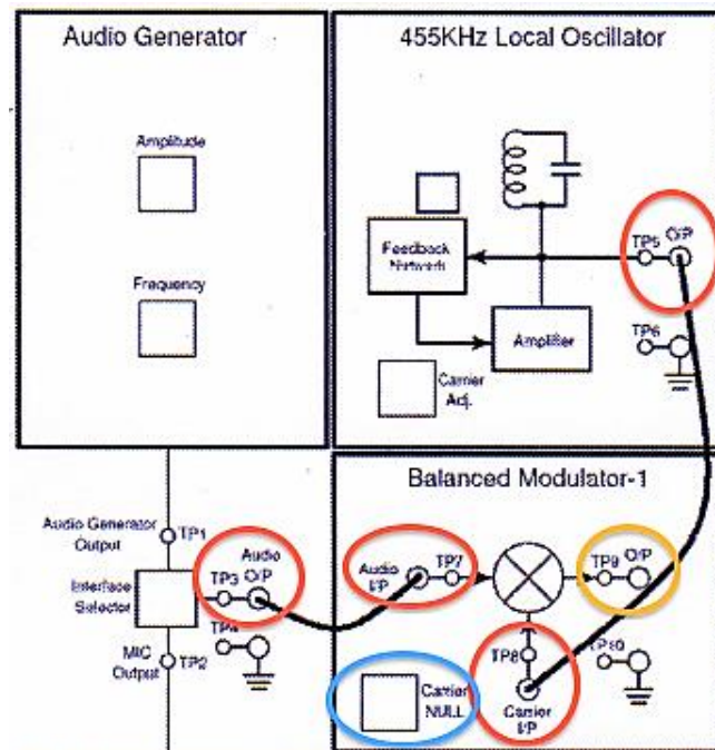
Εικόνα 5 – Συνδεσμολογία πειραματικής διάταξης της υπό εξέταση διαμόρφωσης
