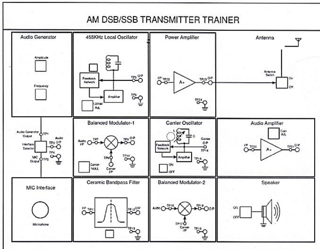
Εικόνα 2 – Σχηματικό διάγραμμα λειτουργικών μονάδων του IT-4101 board
