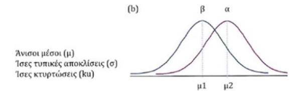
Σχήμα 8.6 - Συμμετρία, άνιση (a) και ίση (b) κύρτωση 2 κατανομών
