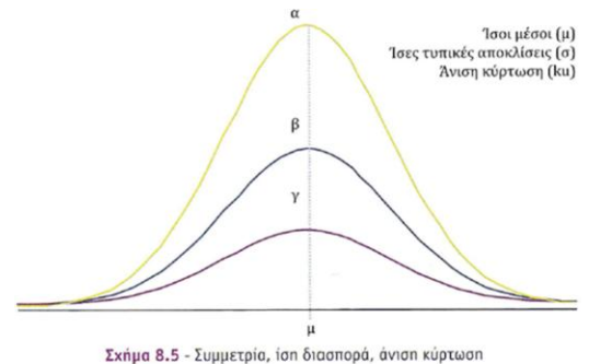
Σχήμα 8.5 - Συμμετρία, ίση διασπορά, άνιση κύρτωση
