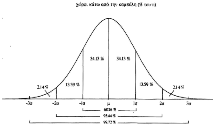
Εικ. 8.3 - Κανονική καμπύλη : κατανομή %f κατά \sigma
