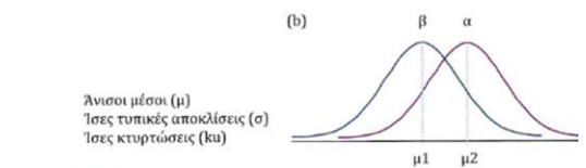
Σχήμα 8.6 - Συμμετρία, άνιση (a) και ίση (b) κύρτωση 2 κατανομών
