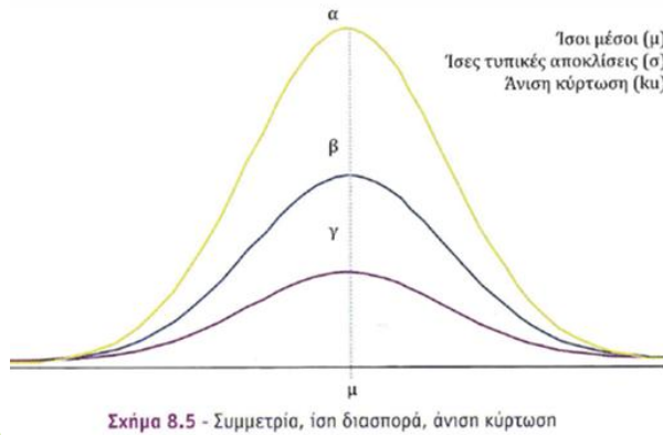
Σχήμα 8.5 - Συμμετρία, ίση διασπορά, άνιση κύρτωση
