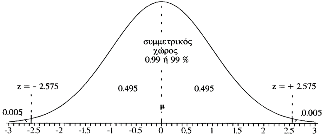
Συμμετρικός χώρος 0.99 της κανονικής καμπύλης
