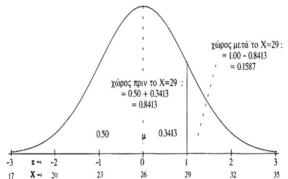
Εικ. 8.9- Χώροι κανονικής καμπύλης πριν & μετά την τιμή z=1
