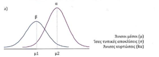
Σχήμα 8.5 - Συμμετρία, ίση διασπορά, άνιση κύρτωση
