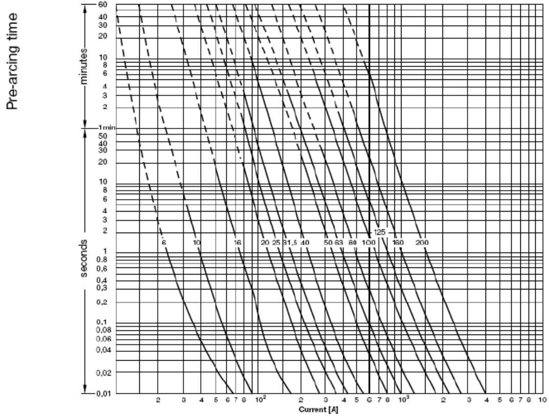
Χαρακτηριστική καμπύλη ασφάλειας σκόνης
